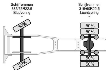
Mercedes-Benz Actros 1846
