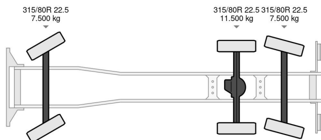
DAF CF 75 250 FAN + Geesink garbage + Krane HIAB 195 6x2
