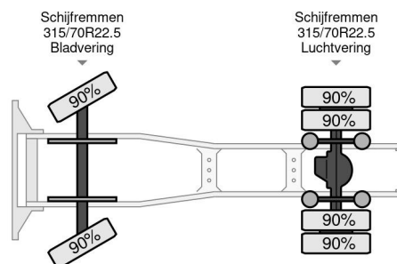
Mercedes-Benz Actros ACTROS F 1945 ADR
