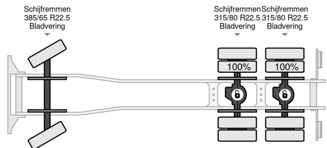
DAF CF 480 FAT + Crane FASSI F235A.2.23 E-DYNAM... 6x4
