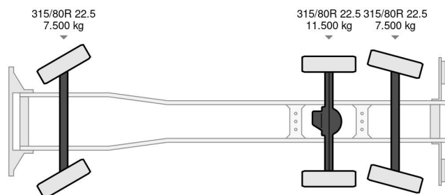
DAF CF 75.250 DAF FAN CF 75 250 + Geesink opbo... 6x2
